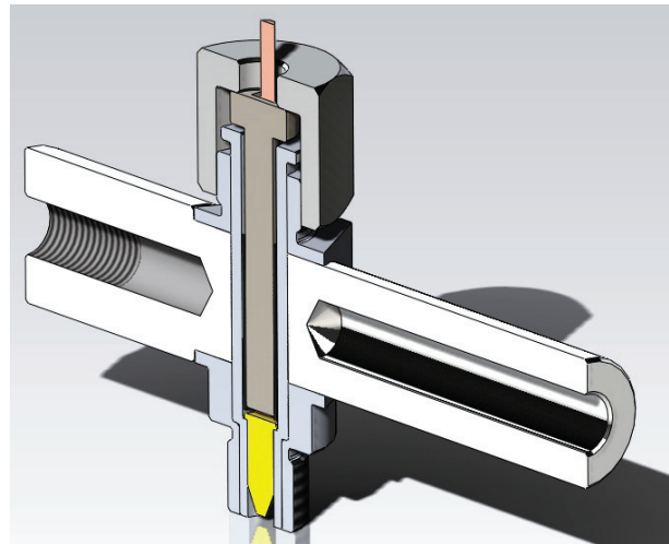
Fig. 3. Blank Ammunition Initiator
