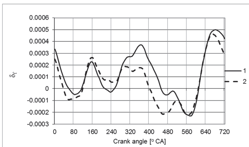
Fig. 11. Values of parameter \delta_f for “strong spring”: 1 – load 250 kW, 2 – load 150 kW
