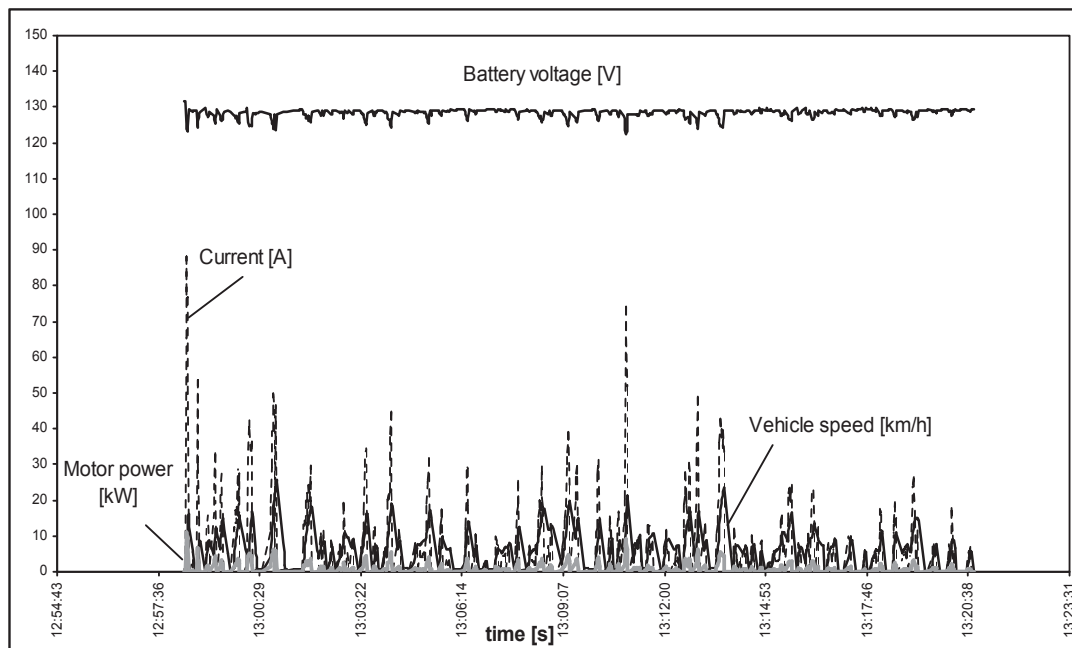
Fig. 10. Stop &amp; go test parameters
