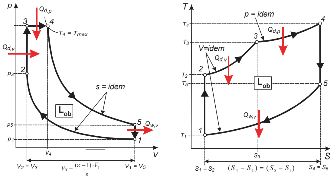
Fig. 3. The Seiliger-Sabathe cycle
