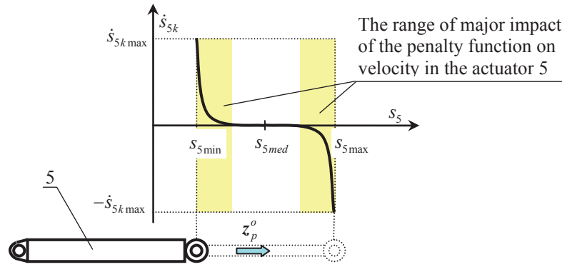
Fig. 3. Penalty function
