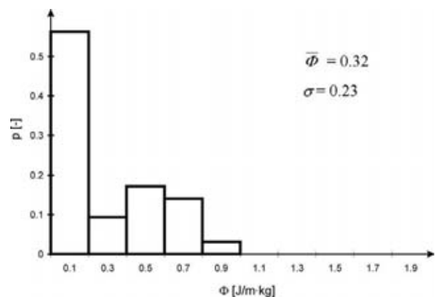
Rys. 8 Histogram rozkładu parametru \Phi (test UDC) Fig. 8 Histogram of parameter \Phi distribution (test UDC)
