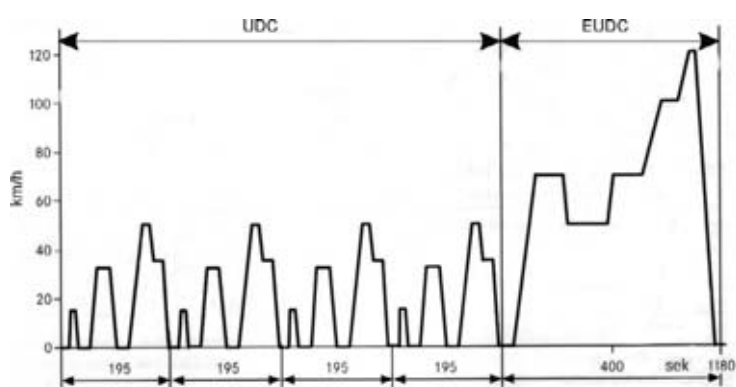
Rys. 1. Przebieg prędkości w teście NEDC [9]
